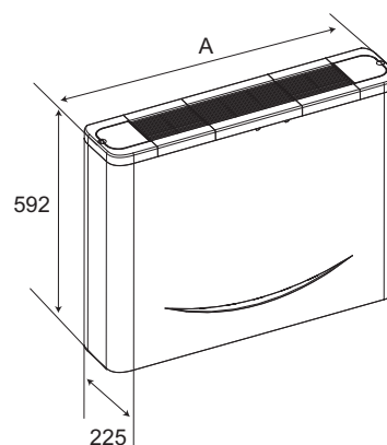
Модель с нижним забором воздуха KP-Izumi II-2P-CB-xx
