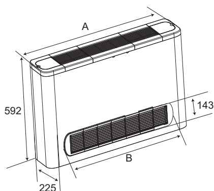
Модель с фронтальным забором воздуха KP-Izumi II-2P-CF-xx
